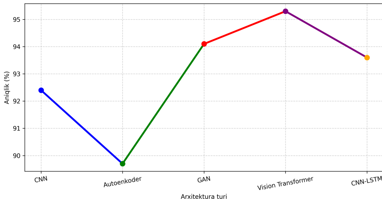
1-rasm. Shaxsga yo'naltirilgan tasvir va videolarga ishlov berishda qo'llaniladigan sun'iy neyron tarmoqlari arxitekturalarining aniqlik ko'rsatkichlari taqqoslanishi 1
