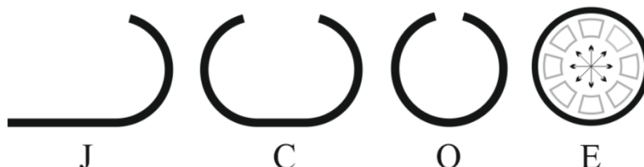
Рисунок 5. Постепенная формовка трубной заготовки штампами 5 (JCOE)
