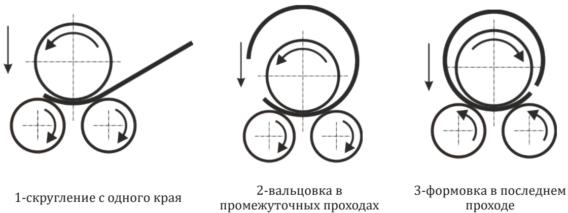
Рисунок 3. Формовка на трех вальцах 3
