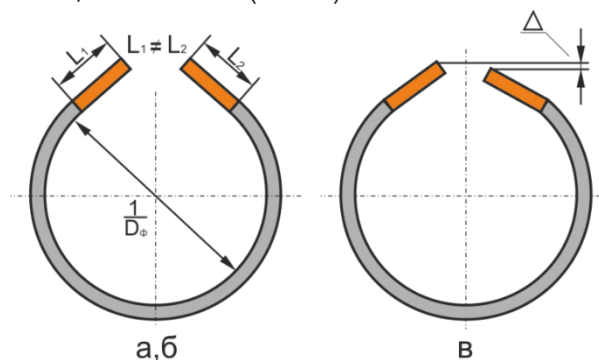
Рисунок 4. Дефекты трубной заготовки при вальцовой формовке 4 : а – плоские кромки, б – неравные длины кромок, в – недоформовка краев
