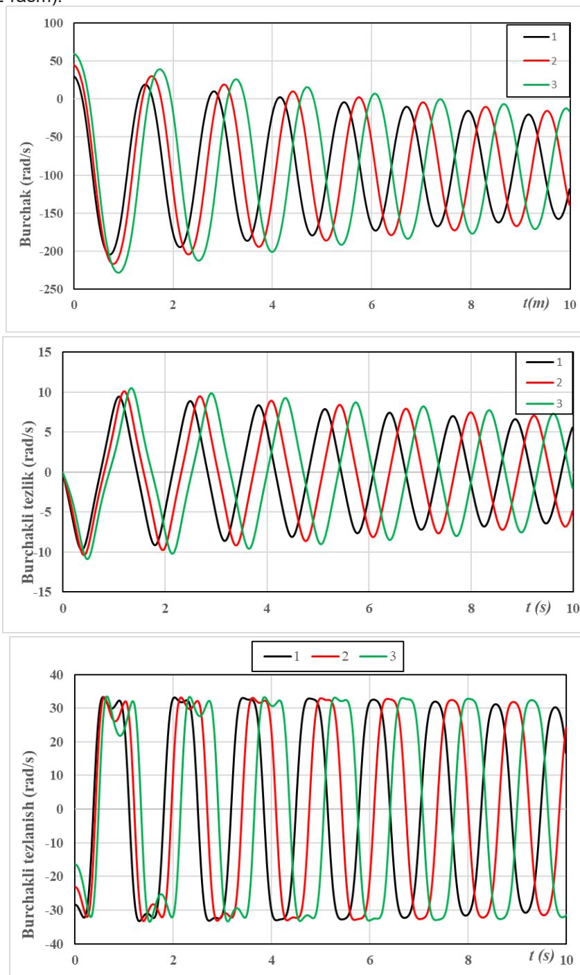
2-rasm. Paxta bo'lagining burchak holati, burchakli tezligi va burchakli tezlanishining vaqtga bog'liqligi ko'rsatilgan.
