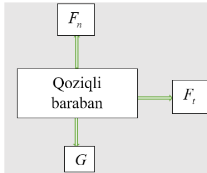
1-rasm. Uzun qoziqli barabanga urilgan paxta bo'lagiga ta'sir etuvchi kuchlar sxemasi
