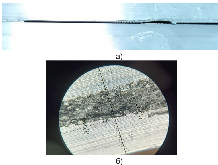
Рис. 1. а) отбракованный профиль с вырезом; б) инородное включение, предположительно ставшее причиной продольного выреза профиля
