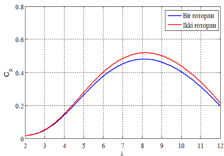
1-rasm. Bir va ikki rotorli shamol turbinasining C_p(\lambda, \beta) quvvat koeffitsiyentini solishtirish
