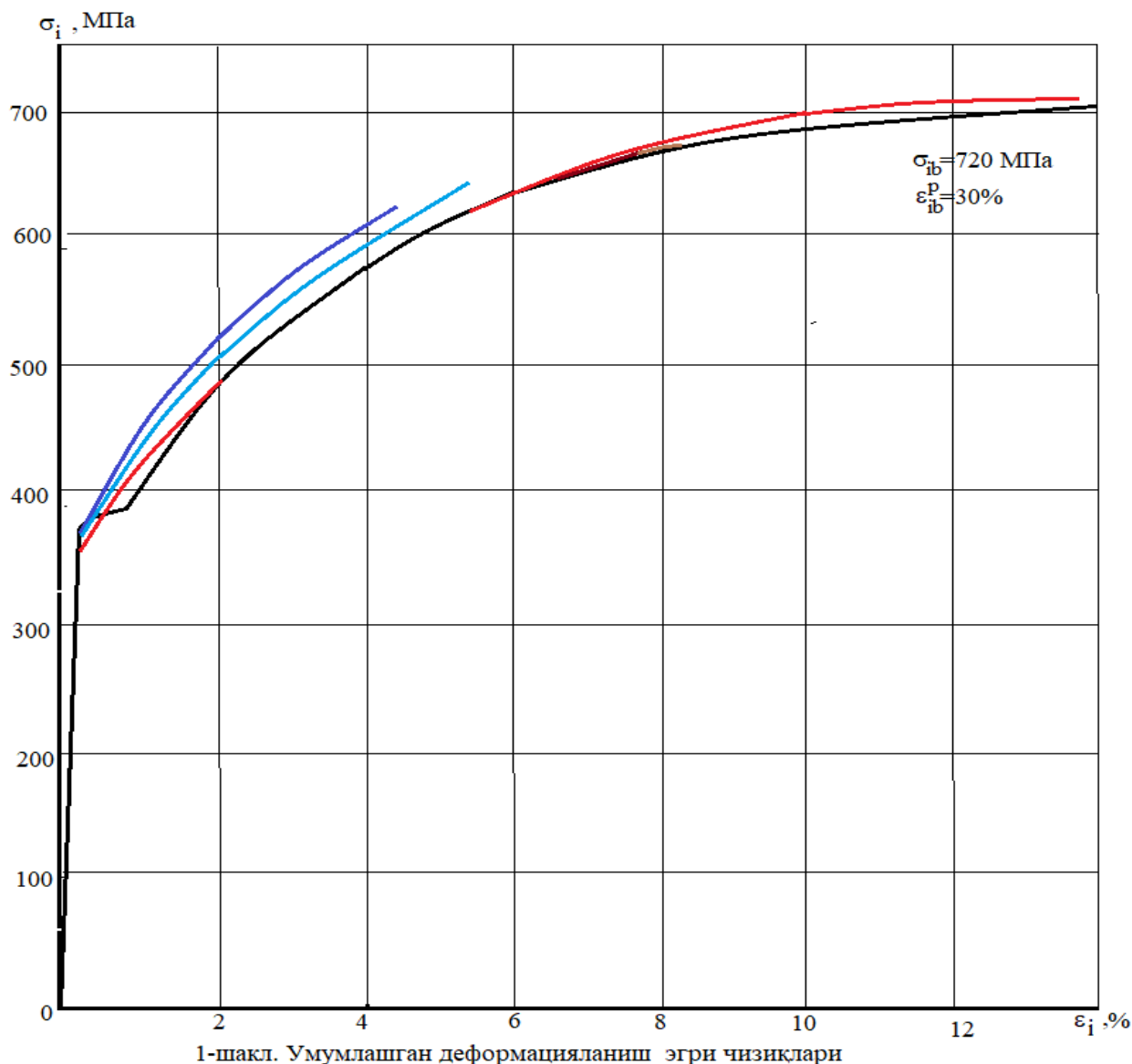
1-rasm. Umumlashgan deformatsiya jarayonining \sigma - \epsilon diagrammalari
