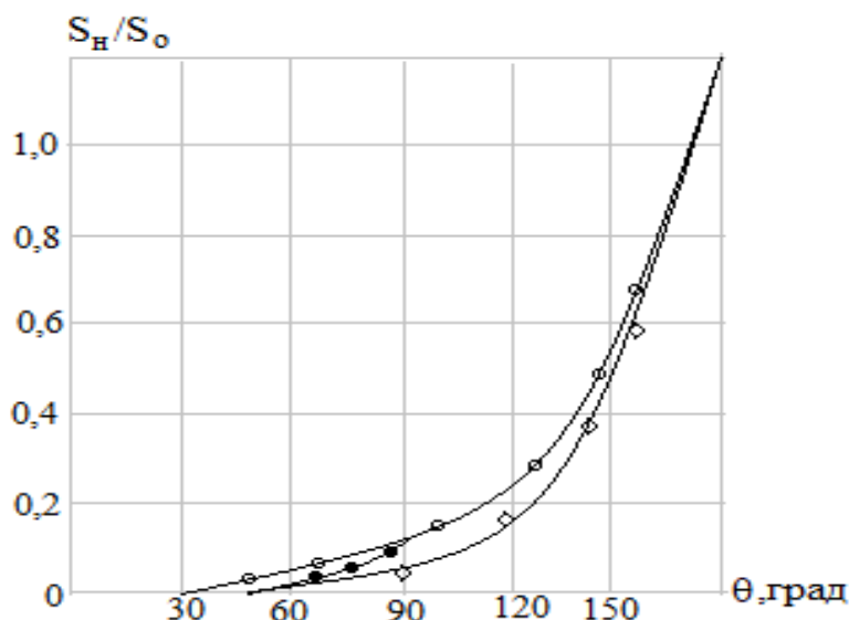
5-шакл. Кучланиш вектори S_H модулини S_0 кучланишга нисбатининг синини бурчагига боғлиқлиги
