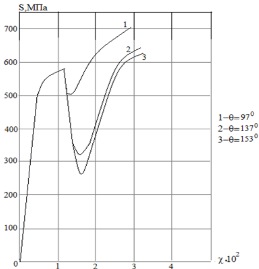
4-shakl. Kuchlanishlar vektori modulinin deformatsion traektoriyasi \theta ni uzundigiga bog'liqligi
