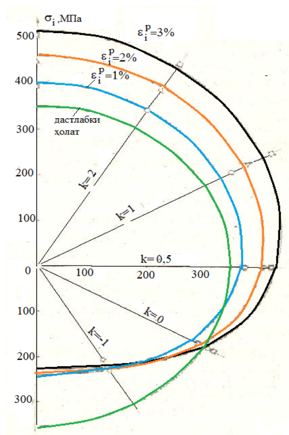
3-шакл. Материалнинг дастлабки ва кейинги оқувчанлик эгри чизиклари
