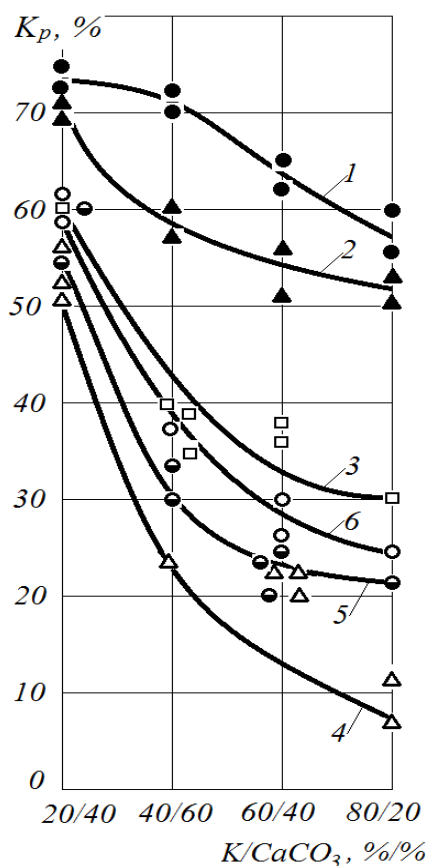
Рис. 3. Зависимость рафинирующей способности флюсов от их состава.
