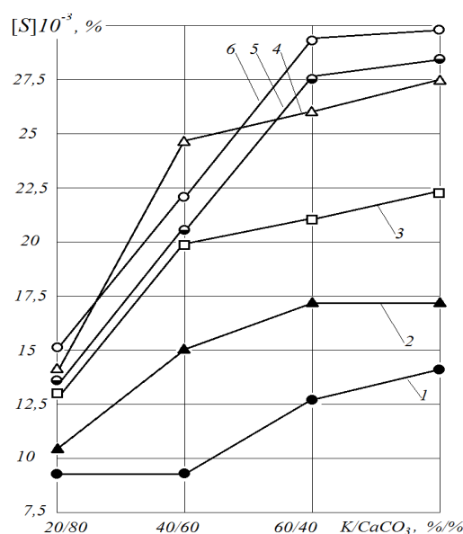
Рис. 2. Зависимость концентрации серы в металле шва от состава шлакообразующей основы флюсов:
