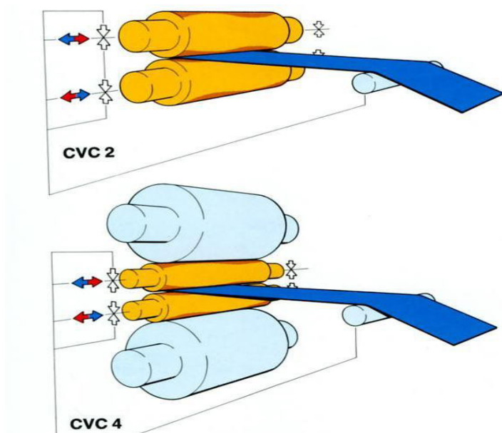
1-rasm. Tasmali listlarni prokatlash sxemasi
